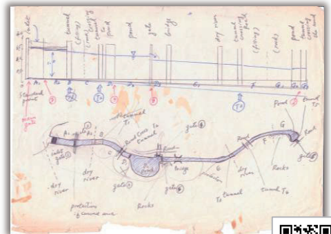
[A-G]用水路概略図 縦断・平面図(2003)
