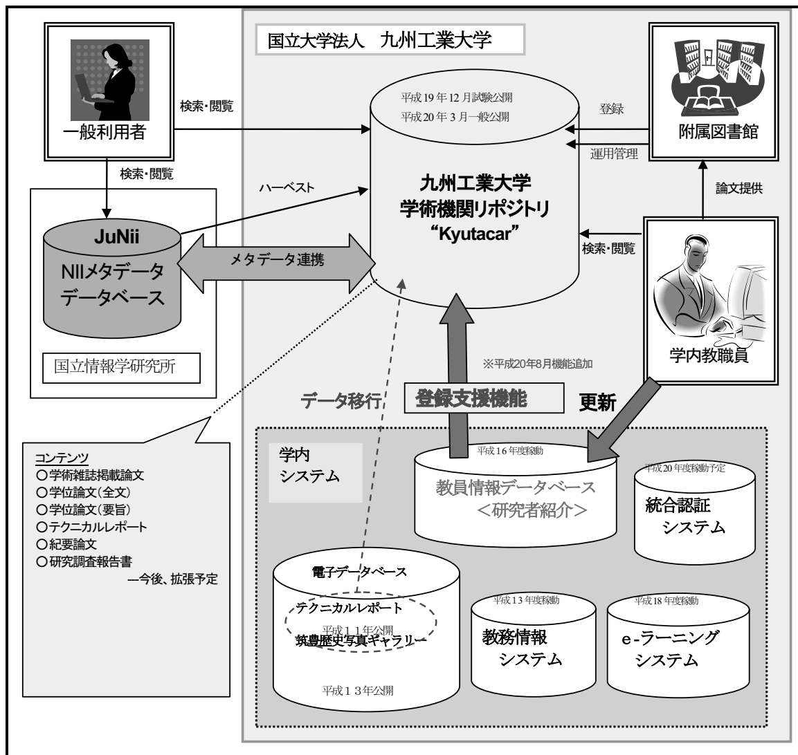
図2 九州工業大学 学術機関リポジトリ構築概念図 (2007年度申請当時)
